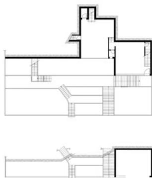
Figura 16a: Abaixo, planta do nível Garagem e acima, planta do nível Vestíbulo e Recreio.
