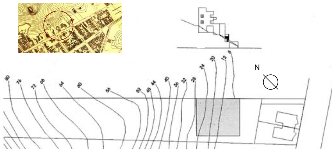
Figura 15a: Levantamento planialtimétrico de 1935.
